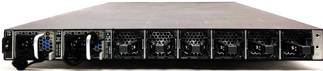
Figure 3 FPR 4112, FPR 4115, FPR 4125, FPR 4145 - Back Panel
