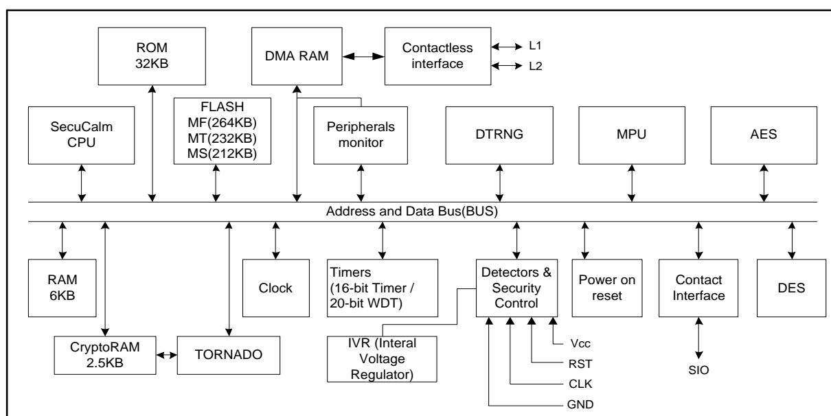
Figure 1 S3FT9MF/S3FT9MT/S3FT9MS Block Diagram
