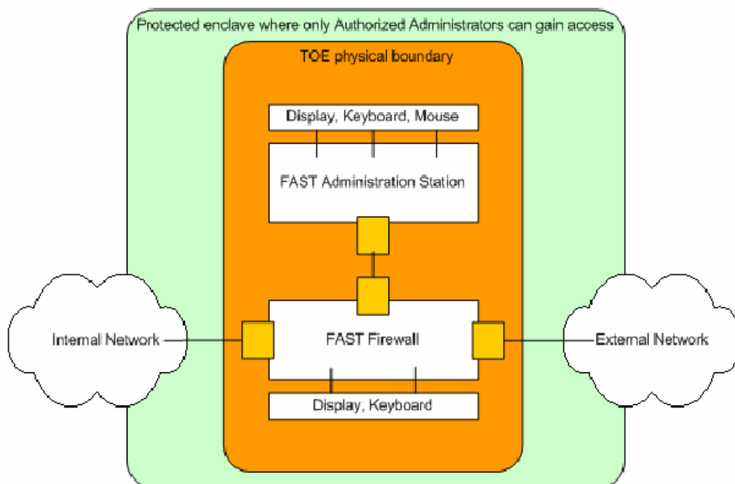
Figure 1 - Périmètre du produit évalué
